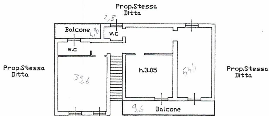
PIANO PRIMO
